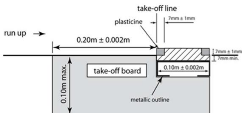
شکل ۹: تخته پرش با تخته سفید
